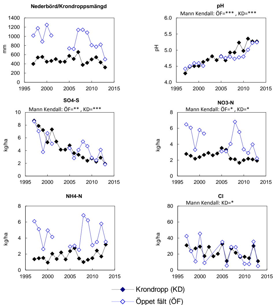
Figur B1:3. Årliga värden (hydrologiskt år) för depositionen via krondropp (KD) och över öppet fält (ÖF) vid Tagel, G22 . Mätplatsen för krondropp flyttades en kortare sträcka 2007. I figuren visas uppmätt nederbörd över öppet fält samt krondroppsmängder, uttryckt som mm. Deposition sedan mätningarna påbörjades redovisas för ett urval av ämnen: pH; sulfatsvavel utan havssaltsbidrag (SO 4 -S ex), nitratkväve (NO 3 -N), ammoniumkväve (NH 4 -N) och klorid (Cl). Trendanalys har genomförts med hjälp av Mann-Kendall analys och signifikansnivåer anges, ovanför respektive diagram, i de fall där signifikanta trender påvisats.
