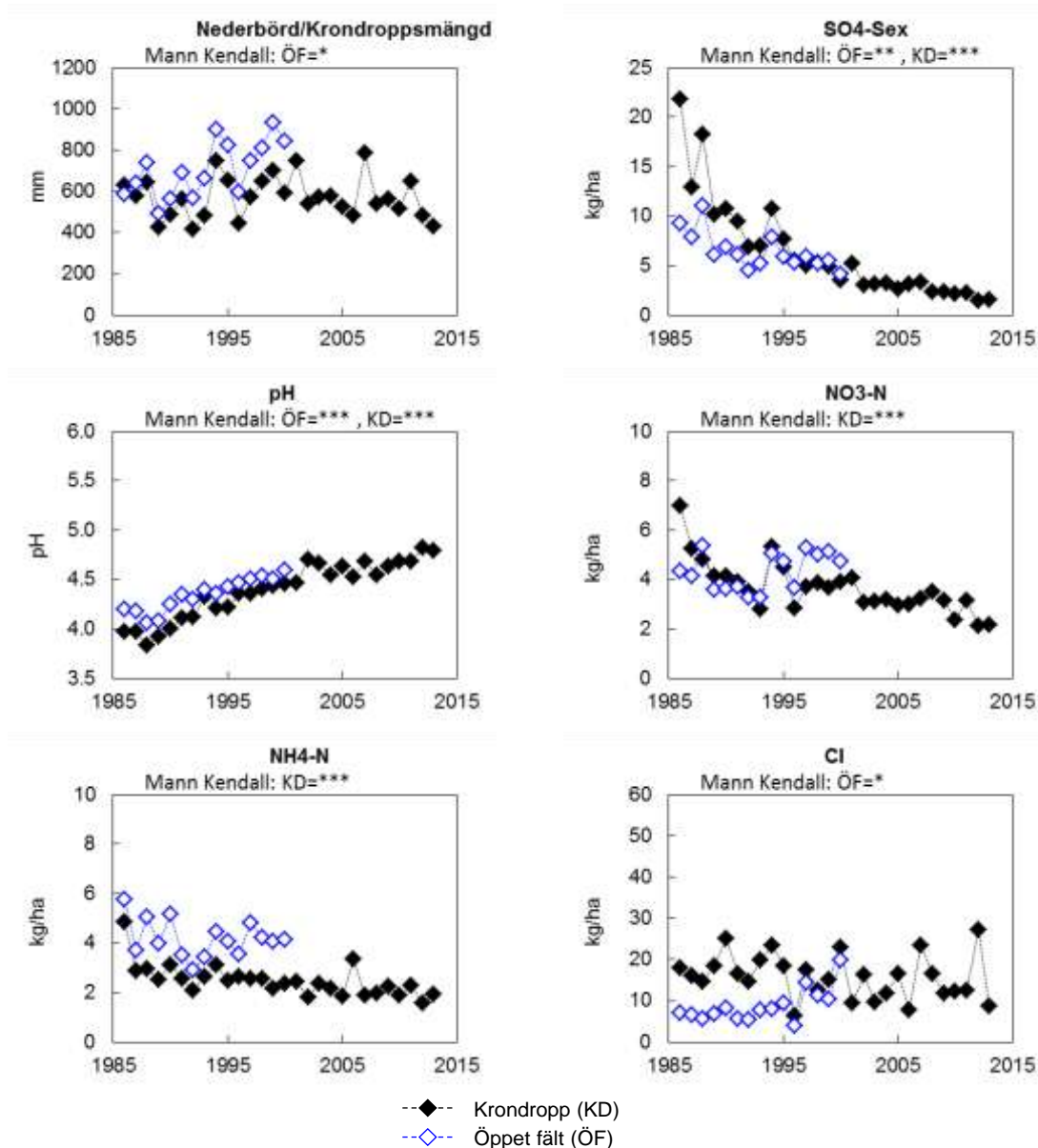
Figur B1:7. Årliga värden (hydrologiskt år) för depositionen via krondropp (KD) och över öppet fält (ÖF) vid Hjärtssjömåla, K 03. I figuren visas uppmätt nederbörd över öppet fält samt krondroppsmängder, uttryckt som mm. Deposition redovisas sedan mätningarna påbörjades för ett urval av ämnen: sulfatsvavel utan havssaltsbidrag (SO4-S ex); pH; nitratkväve (NO3-N); ammoniumkväve (NH4-N) och kloridjoner (Cl-). Trendanalys har genomförts med hjälp av Mann- Kendall metodik och signifikansnivåer anges, ovanför respektive diagram, i de fall där signifikanta trender påvisats.
