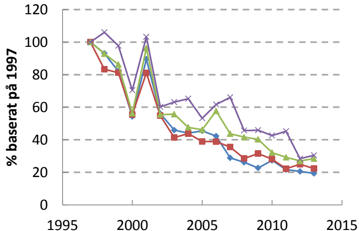
Figur 3. Årliga värden för nedfall av sulfatsvavel till tre platser i Kronobergs län, samt en närliggande mätplats med tallskog i Blekinge län (Hjärtsjömåla) uppmätt som krondropp, i absoluta tal (A) och som procent utgående från året 1997 (B). Nedfallet i krondropp mättes månadsvis och summerades för hydrologiskt år (okt-sept).
