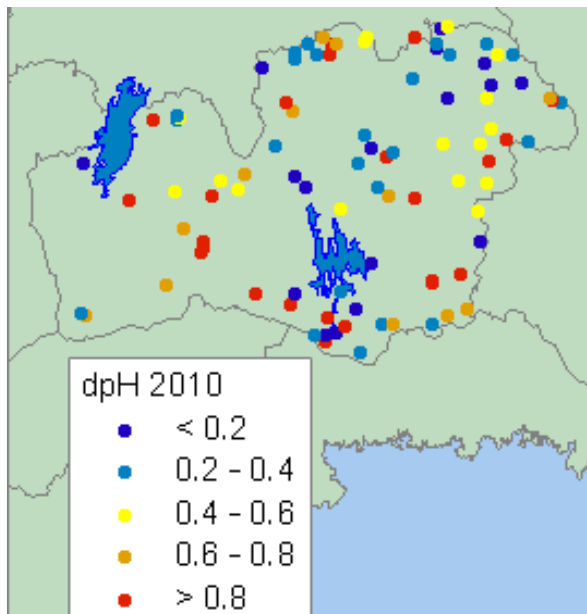
Figur 7. pH-förändring sedan förindustriell tid (dpH) i sjöar 2010, baserat på MAGIC-biblioteket. En sjö räknas som antropogent försurad om pH som årsmedian har sjunkit med minst 0,4 enheter sedan förindustriell tid (dpH > 0,4), vilket markeras med gula, orange och röda symboler på kartan
