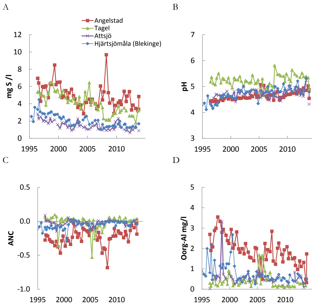
Figur 5. Halterna av sulfatsvavel (A, SO 4 -S), pH (B), syraneutraliserande förmåga (C, ANC) och halten oorganiskt aluminium (D, oorg-Al) i markvattnet på 50 cm djup vid olika platser i Kronobergs län, uppmätt inom Krondropps nätet. Följande förändringar är statistiskt säkerställda: Halterna av SO 4 -S har minskat signifikant vid alla mätplatser; pH och ANC har ökat och oorganiskt aluminium har minskat signifikant vid Angelstad.
