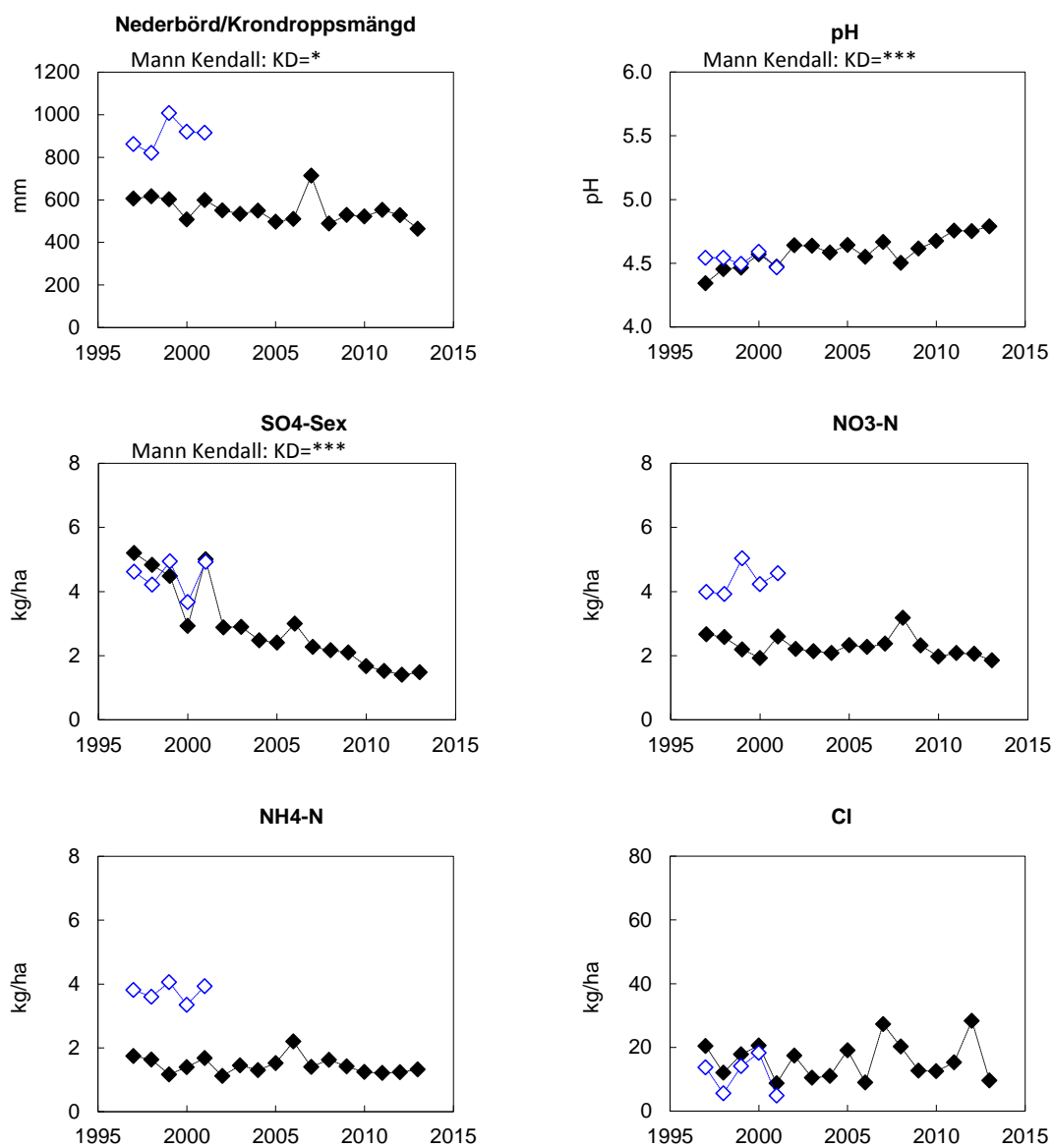
Figur B1:1. Årliga värden (hydrologiskt år) för depositionen via krondropp (KD) och över öppet fält (ÖF) vid Attsjö, G21 . I figuren visas uppmätt nederbörd över öppet fält samt krondroppsmängder, uttryckt som mm. Deposition sedan mätningarna påbörjades redovisas för ett urval av ämnen: pH; sulfatsvavel utan havssaltsbidrag (SO 4 -Sex), nitratkväve (NO 3 -N); ammoniumkväve (NH 4 -N) och kloridjoner (Cl). Trendanalys har genomförts med hjälp av Mann-Kendall analys och signifikansnivåer anges, ovanför respektive diagram, i de fall där signifikanta trender påvisats.
