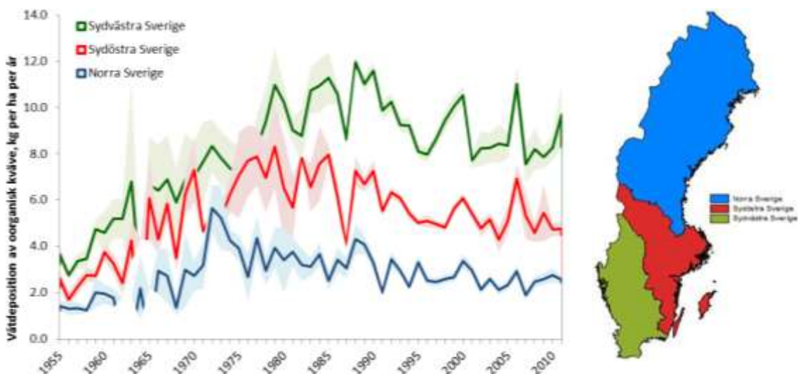
Figur 13. Nedfallet av oorganiskt kväve (NO 3 + NH 4 ) med våtdepositionen (kg/ha/år) i tre regioner (se karta) för åren 1955-2011. Utöver våtdepositionen finns ett litet inslag av torrdeposition från provtagningsutrustningen I provet. Linjerna visar årsvisa medelvärden från de lokaler som det finns mätdata från det aktuella året. Det färgade området kring linjerna visar medelfelet i data (Standard Error). Det är olika antal stationer olika år. Man ser att variationen i data minskade efter det att Krondroppsnetet startade 1985 främst på grund av att antalet mätstationer ökade. Efter 2003 har antalet mätplatser återigen minskat. Källa: IVL, 2013; Hansen m.fl., 2013.
