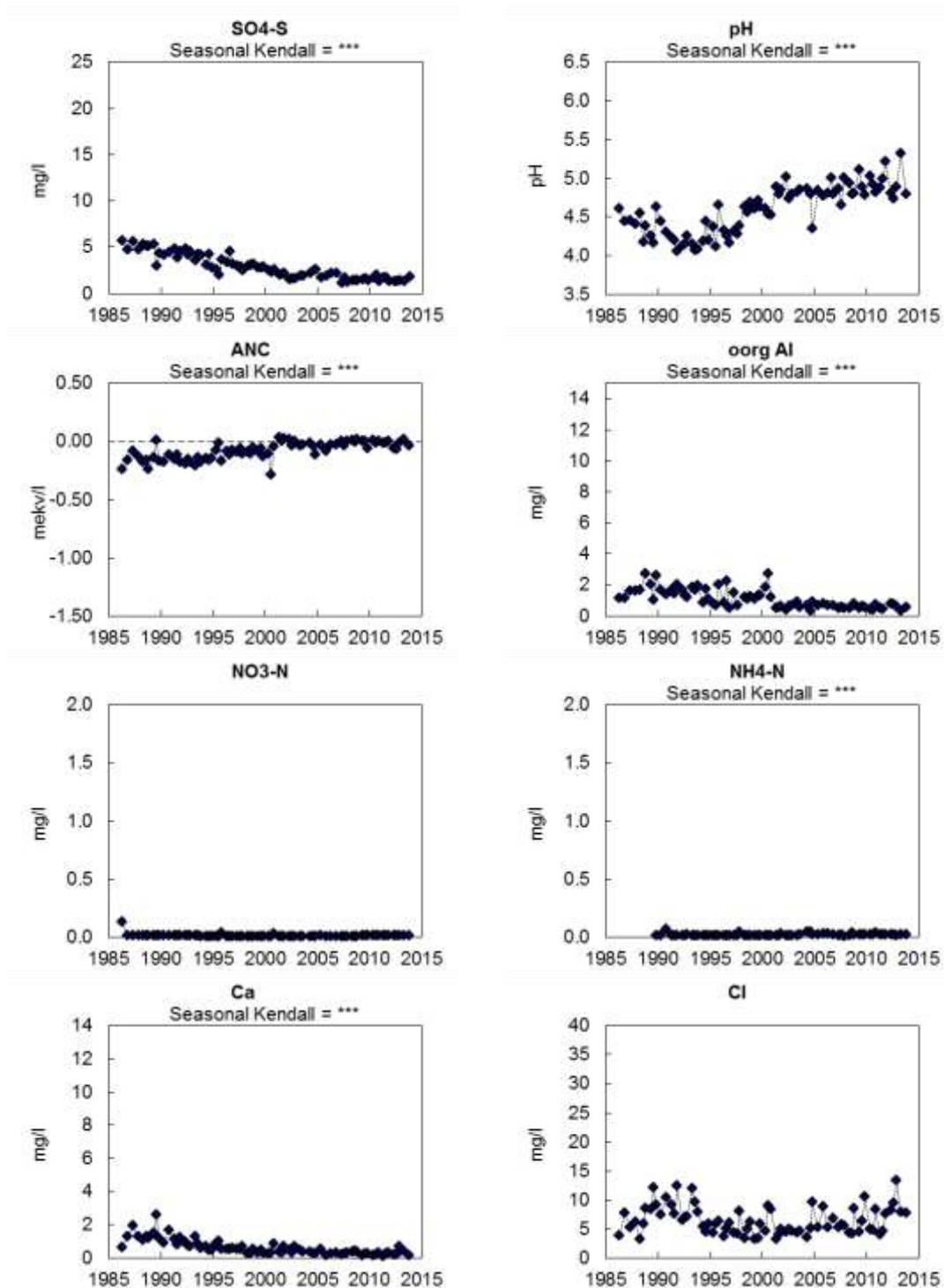
Figur B1:8. Markvattenkemi vid Hjärtsjömåla, K 03 . Sulfatsvavel (SO 4 -S); pH; markvattnets syraneutraliserande förmåga (ANC); oorganiskt aluminium (oorg Al); nitratkväve (NO 3 -N); ammoniumkväve (NH 4 -N); kalciumhalt (Ca 2+ ) och kloridhalt (Cl). Saknade värden innebär oftast att marken varit för torr. Trendanalys har genomförts med hjälp av Seasonal-Kendall metodik och signifikansnivåer anges, ovanför respektive diagram, i de fall där signifikanta trender påvisats.
