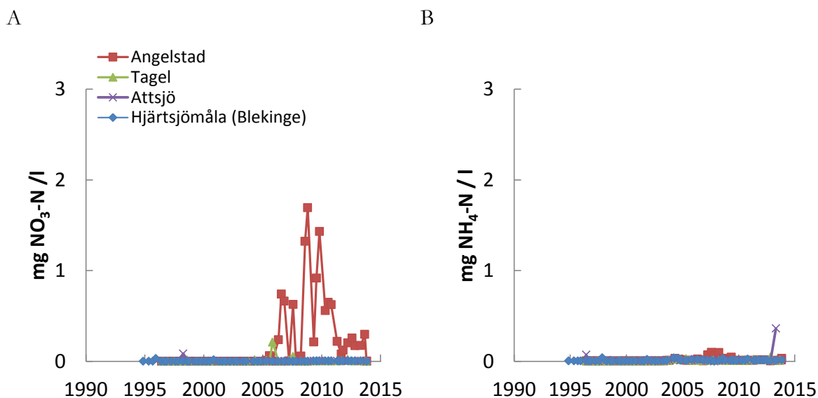
Figur 10. Halterna i markvattnet på 50 cm djup vid olika platser i Kronobergs län av nitratkväve (NO 3 -N) (A) samt ammoniumkväve (NH 4 -N) (B). Inga förändringar är statistiskt säkerställda. För Angelstad finns en statistiskt säkerställd ökning av halterna av nitrat sedan mätningarna startade 1996. Detta har dock sannolikt ett samband med effekterna av stormarna Gudrun och Per samt även senare stormfällan.
