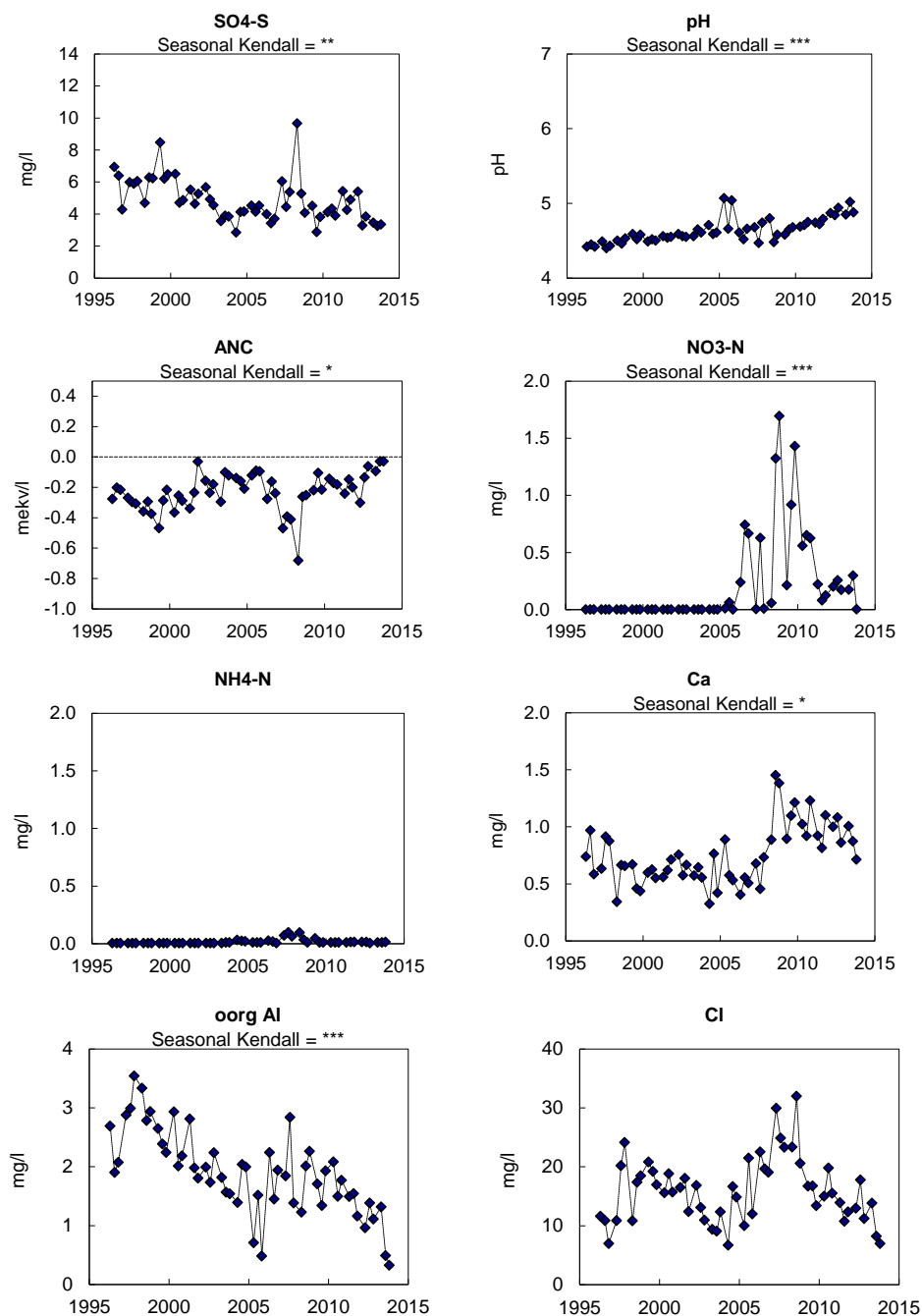
Figur B1:6. Markvattenkemi vid Angelstad, G 23: sulfatsvavel ( \text{SO}_4\text{-S} ), pH, markvattnets syraneutraliserande förmåga (ANC), nitratkväve ( \text{NO}_3\text{-N} ), ammoniumkväve ( \text{NH}_4\text{-N} ), kalciumhalt ( \text{Ca}^{2+} ); oorganiskt aluminium (oorg Al) samt kloridhalt ( \text{Cl}^- ). Saknade värden innebär oftast att marken varit för torr. Trendanalys har genomförts med hjälp av Seasonal-Kendall och signifikansnivåer anges, ovanför respektive diagram, i de fall där signifikanta trender påvisats. Ytan var påverkad av stormarna Gudrun och Per. Dessutom uppstod vid ett antal tillfällen stormfällan även under senare år.
