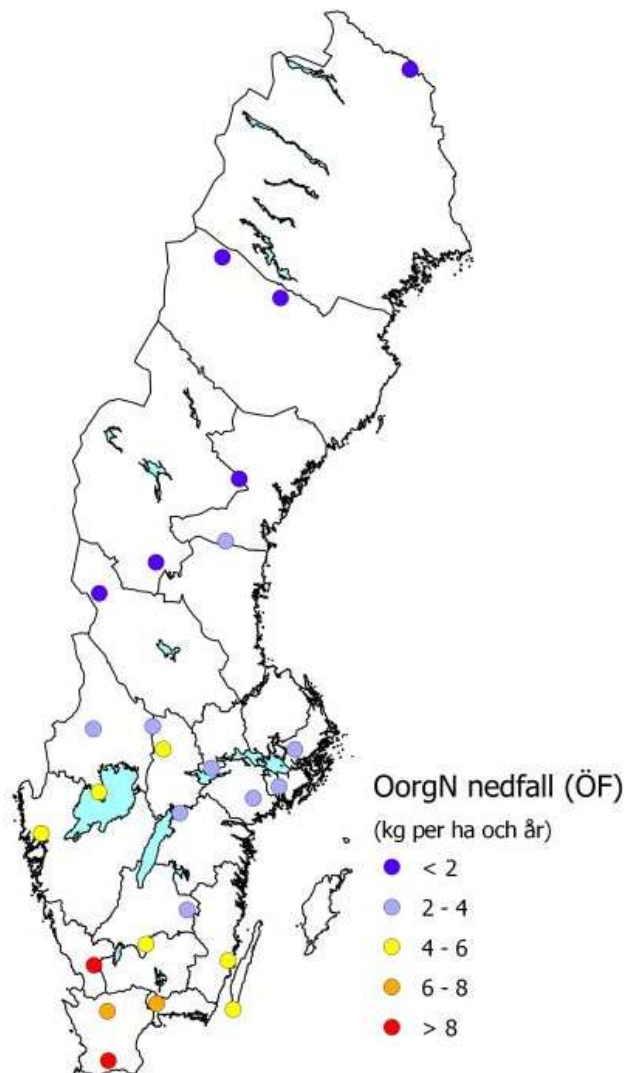
Figur 9. Nedfallet av oorganiskt kväve (oorgN) med nederbörden till öppet fält vid olika platser inom Krondroppsnetet under det hydrologiska året 2013/13.
